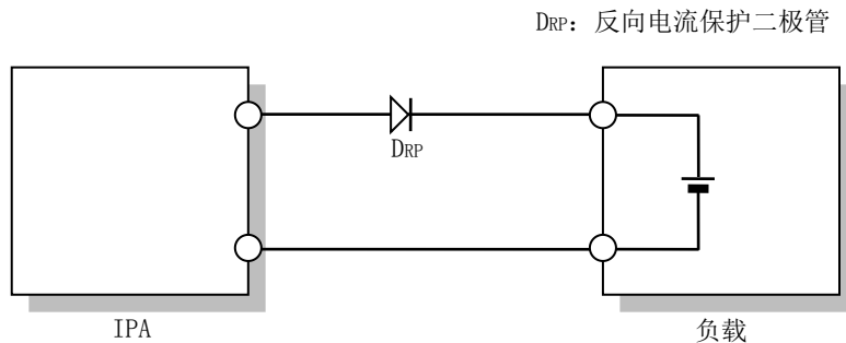
图 3-4 储能负载的连接方法
