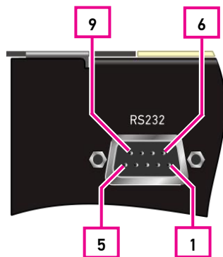
图 5-2 IPL 系列电源 RS232C 接口定义
